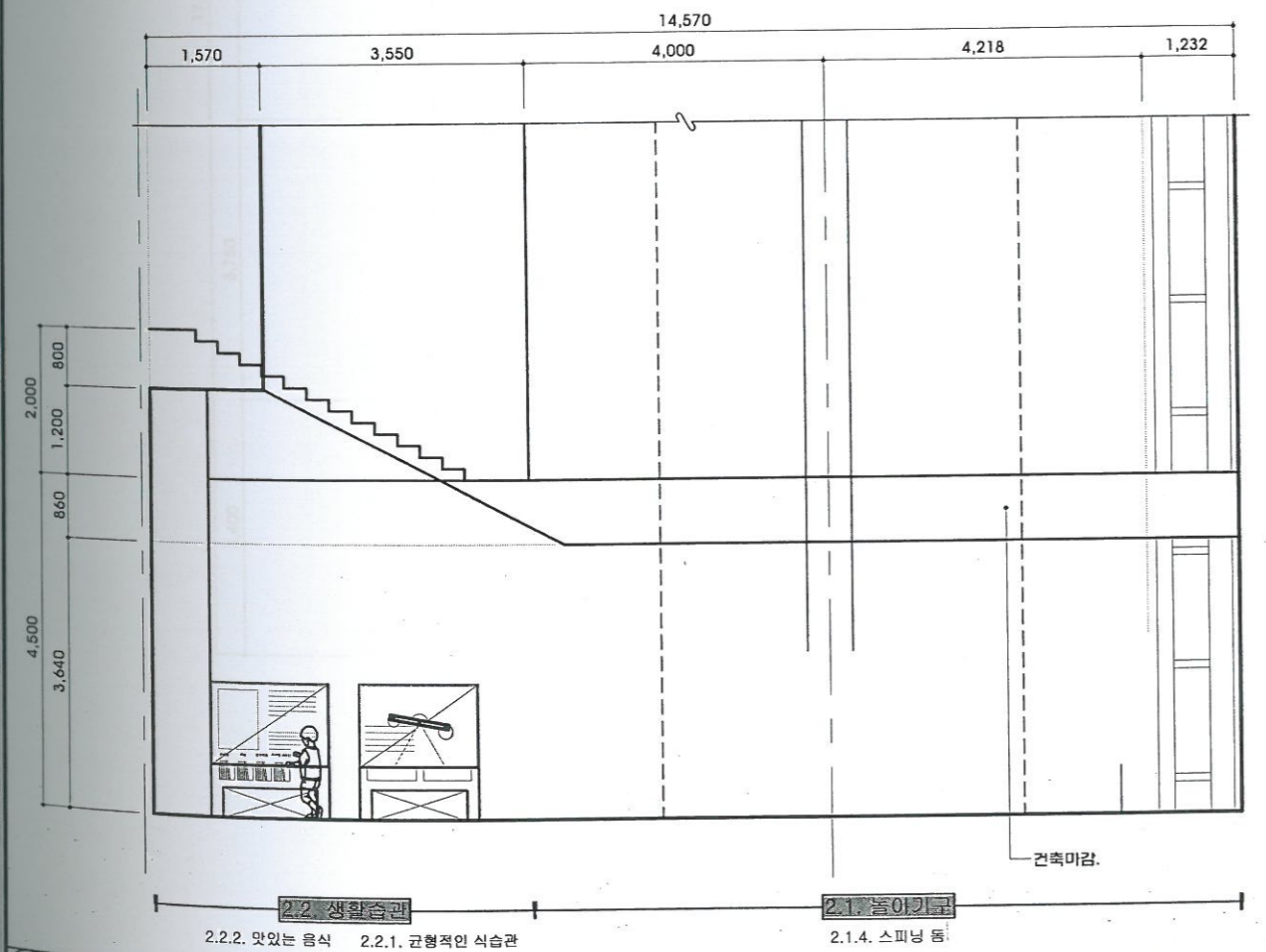
2 Gallery 2. 튼튼 놀이터 입면도-2
