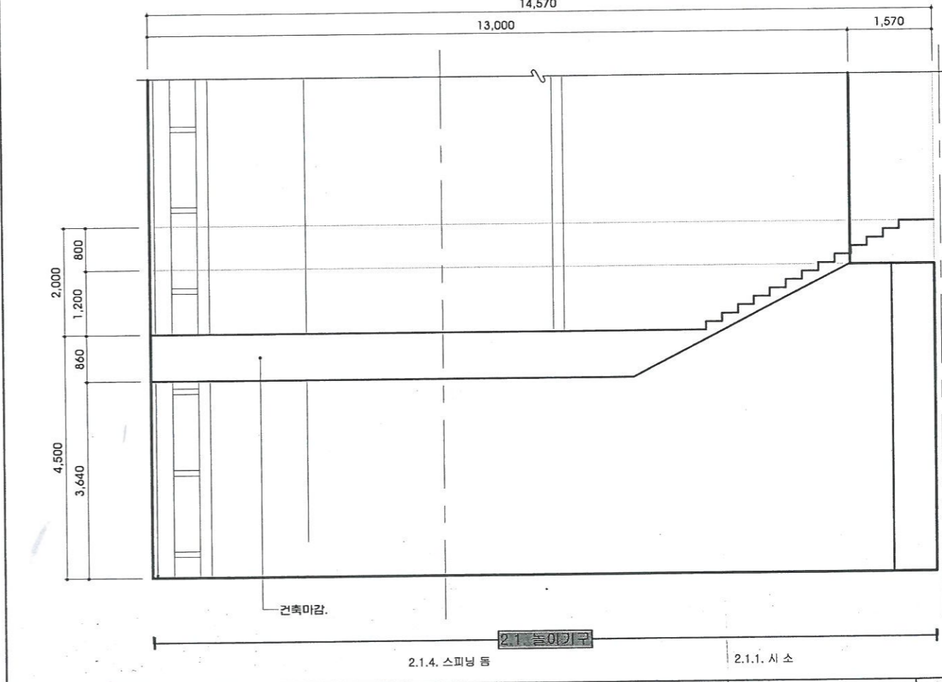
3 Gallery 2. 튼튼 놀이터 입면도-3
